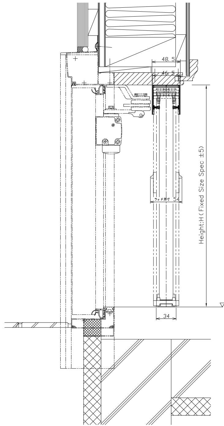
Tenpooh Latch Type Longitudinal section
