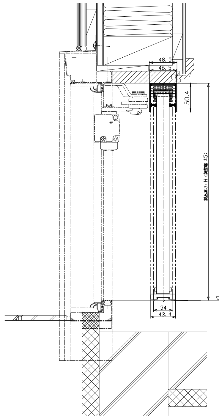
Tenpoo Magnet Type Longitudinal section
