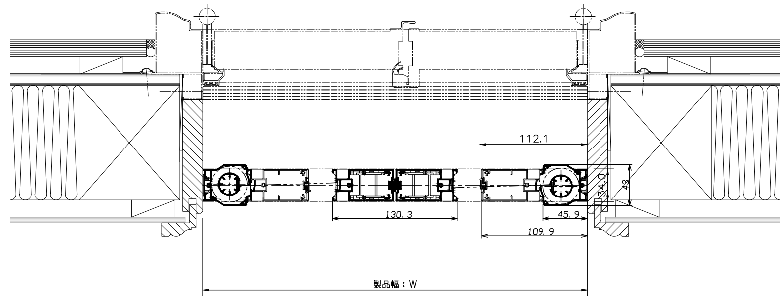
Double door Cross section
