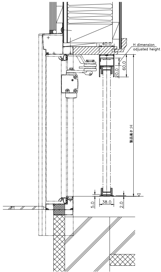
Zipooh (8LME) Longitudinal section
