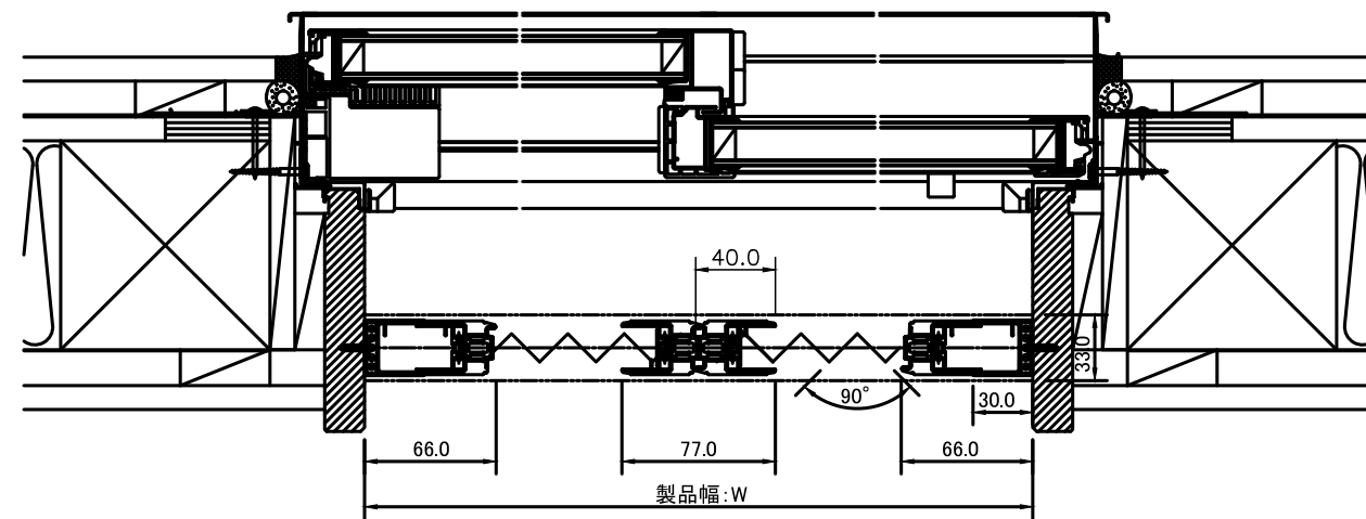
インテリア網戸 側面付 引分け(20mm)横断面図 W/2 < 960 STLSF適用
