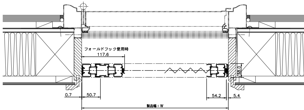
侍風 片引き (88LME) 横断面図
