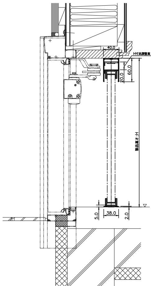
侍風 (88LME) 縦断面図
