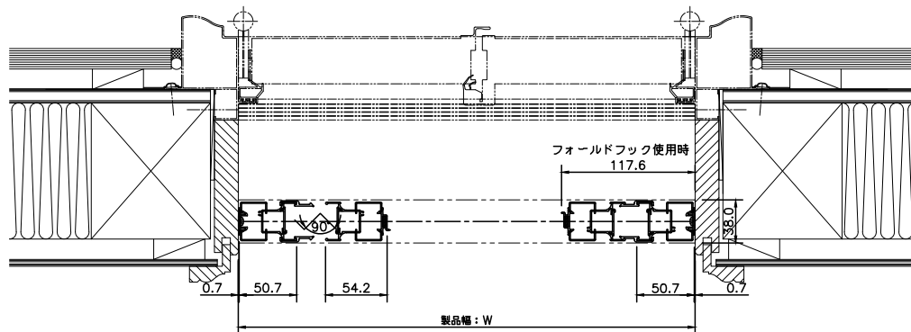
侍風 両引き (88LME) 横断面図
