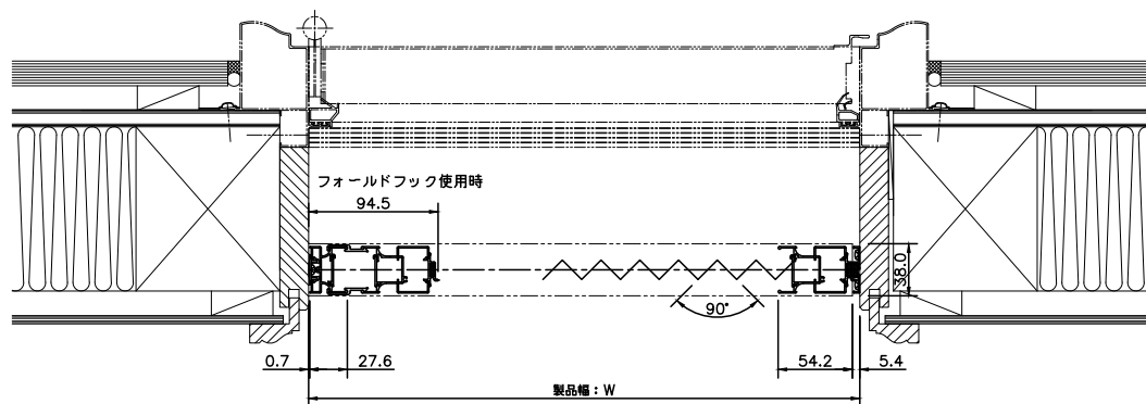
侍風 片引き (8LME) 横断面図
