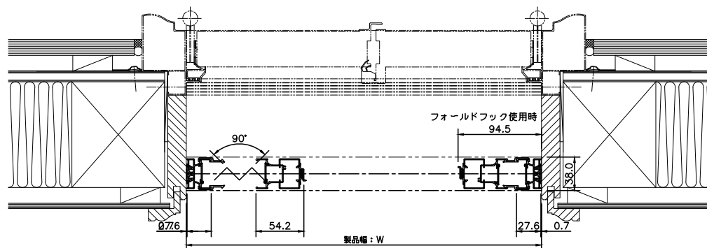
侍風 両引き (8LME) 横断面図
