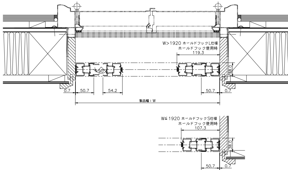
侍風 両引き (88LME) 横断面図
