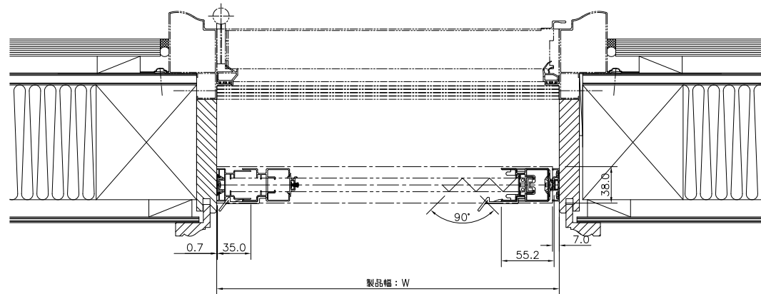
ぎやたぴら網戸2 片引き (8LF) 横断面図
