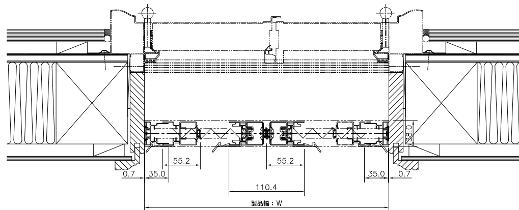
ぎやたぴら網戸2 両引き (8LF) 横断面図
